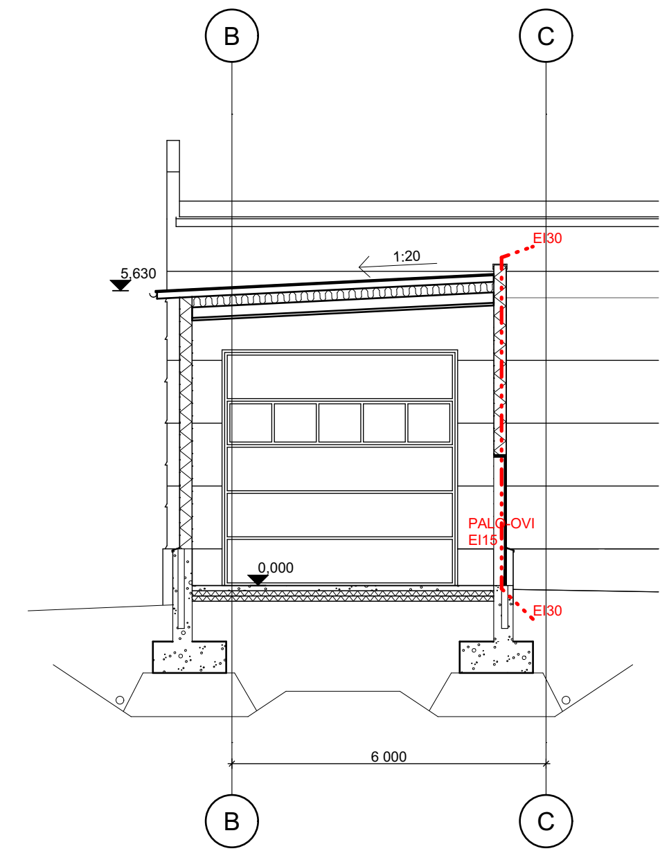
LEIKKAUS B-B
