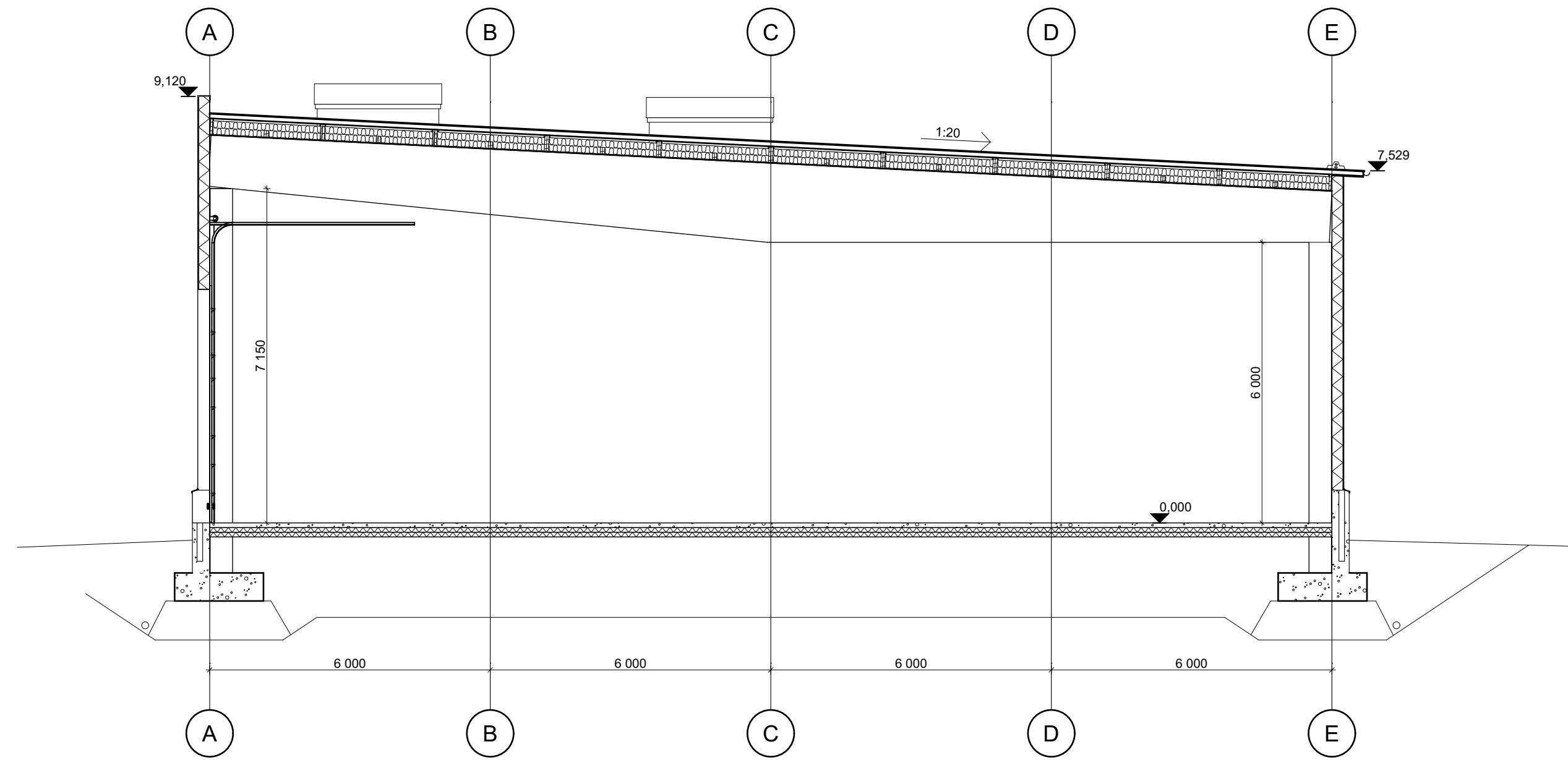
LEIKKAUS A-A
