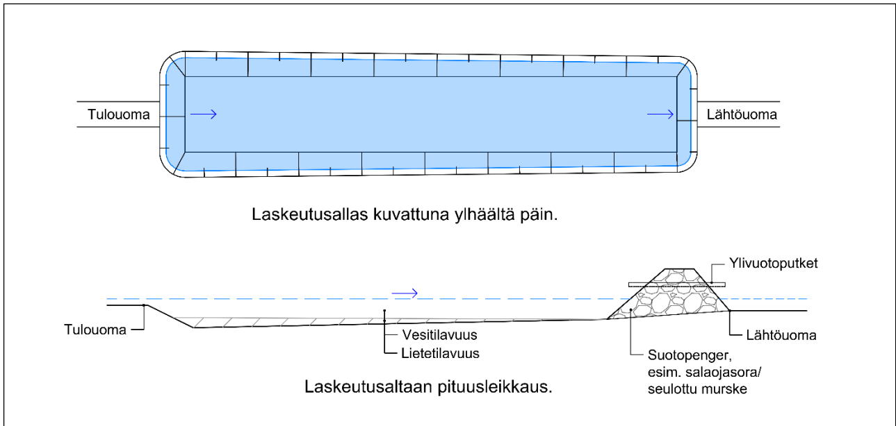
Kuva 8. Purkuojan yhteyteen rakennettavan laskeutusaltaan ja suotopenkereen periaatekuvat.
