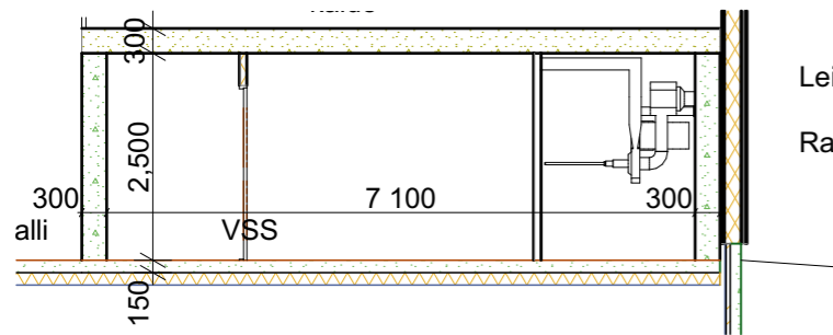
A Leikkaus 1:100
