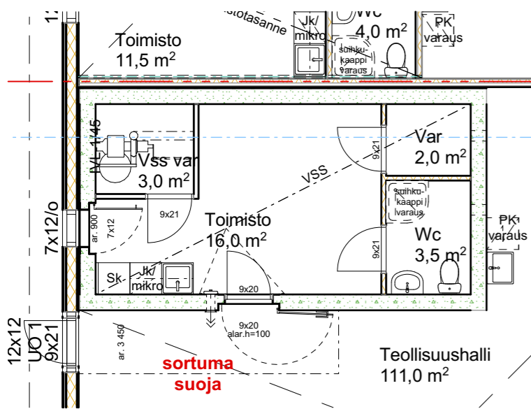
1. kerros 1:100
