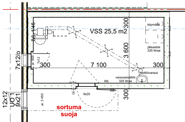
VSS 1:100
